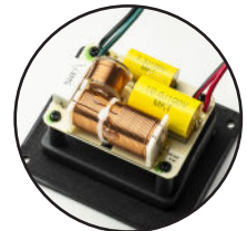
Diskrete Frequenzweiche
